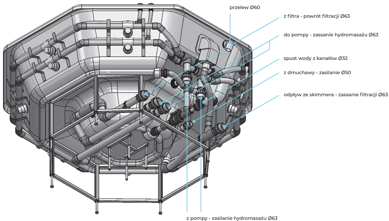
Schemat technologiczny dla wanny SPA ze skimmerem i z podwójnym rzędem dysz na przykładzie wanny Vesta
