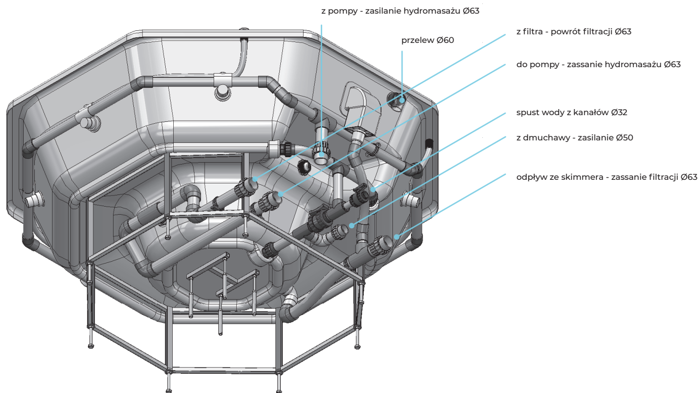
Schemat technologiczny dla wanny SPA ze skimmerem i z pojedynczym rzędem dysz na przykładzie wanny Vesta
